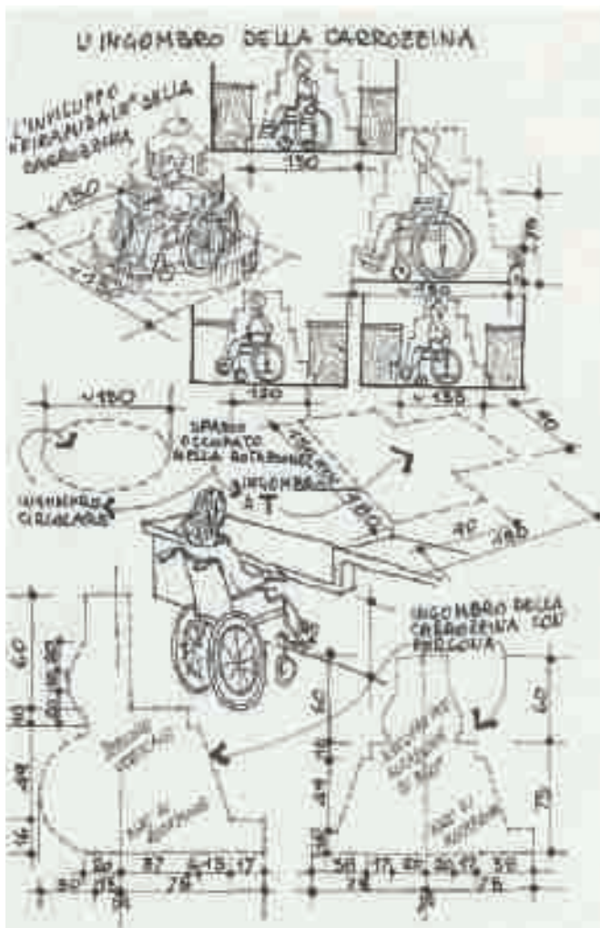
Indicazioni sull'ingombro della carrozzina
